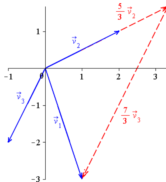
Abbildung 9: \vec{v}_1 = \frac{5}{3}\vec{v}_2 + \frac{7}{3}\vec{v}_3
