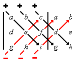
Abbildung 11: Regel von Sarrus
