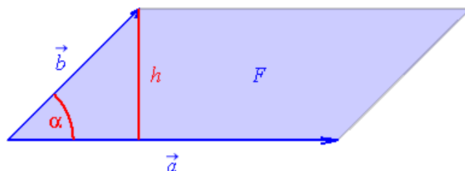
Abbildung 7: \|\vec{a} \times \vec{b}\| entspricht der Fläche des aufgespannten Parallelogramms
