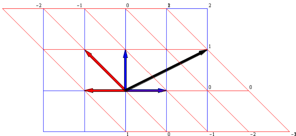
Abbildung 10: Der Vektor \vec{v} (schwarz) bezüglich der Basis E (blau) und bezüglich der Basis B (rot). Es gilt \vec{v} = \begin{pmatrix} 2 \\ 1 \end{pmatrix}_E bzw. \vec{v} = \begin{pmatrix} -3 \\ 1 \end{pmatrix}_B .
