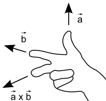
Abbildung 6: Rechte-Hand-Regel und Vektorprodukt
