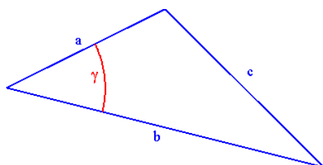
Abbildung 4: a^2 + b^2 - 2ab \cdot \cos \gamma = c^2 (Cosinussatz)
