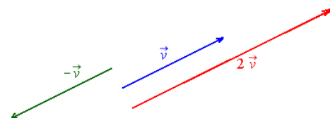
Abbildung 2: Multiplikation eines Vektors mit einem Skalar.
