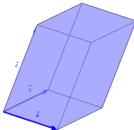
Abbildung 8: |\vec{a} \cdot (\vec{b} \times \vec{c})| entspricht dem Volumen des aufgespannten Spats
