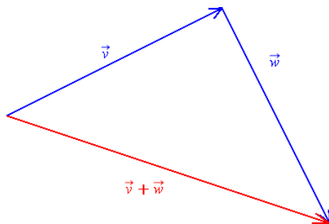
Abbildung 1: Addition von Vektoren.
