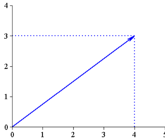
Abbildung 3: \left\| \begin{pmatrix} 4 \\ 3 \end{pmatrix} \right\| = \sqrt{4^2 + 3^2} = 5
