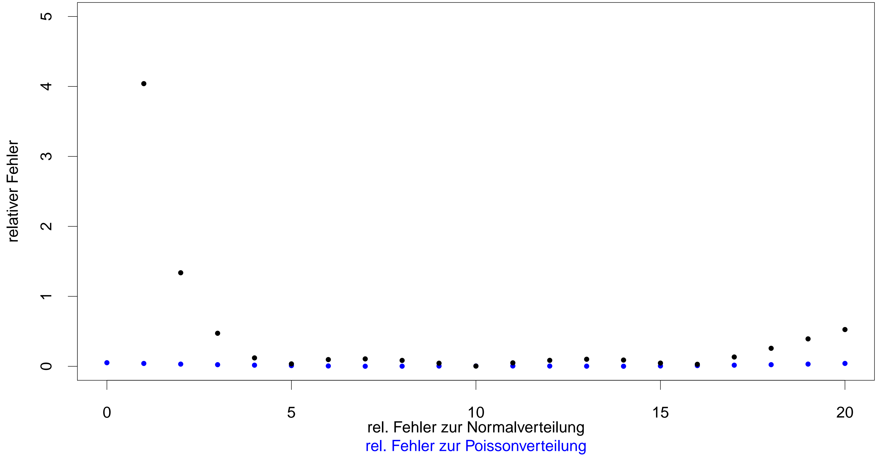
Plot der relativen Fehler k=0,1,\dots,20
